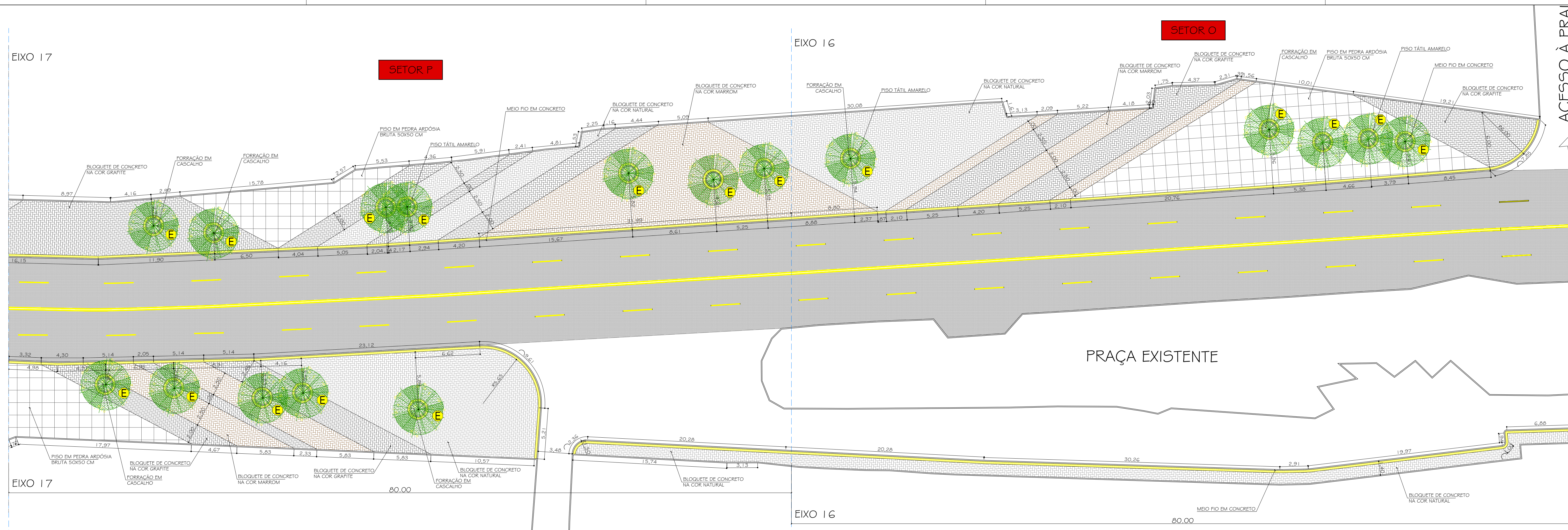
PLANTA BAIXA - ETAPA 6 - SETORES O E P AVENIDA DOS ARRECIFES ESCALA:.....1/200
